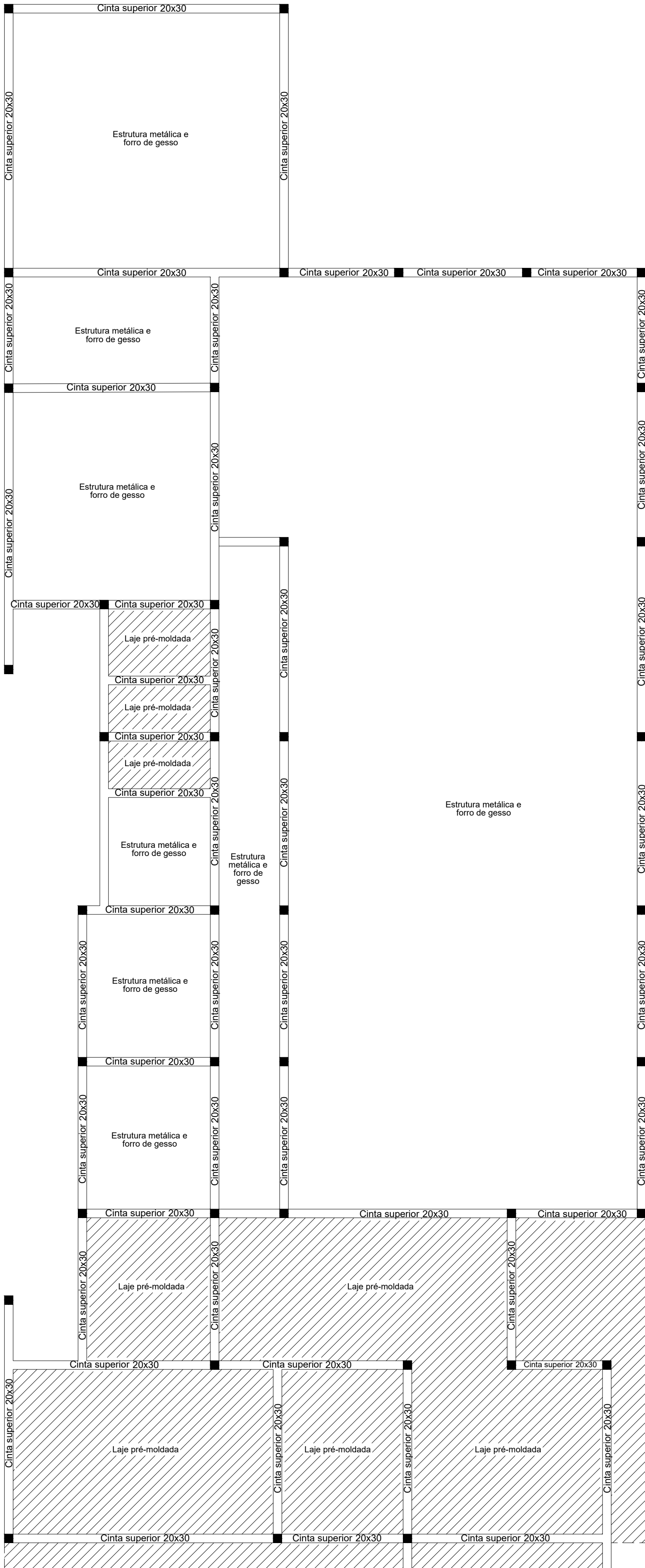
Forma da cinta superior da edificação (3,50)
